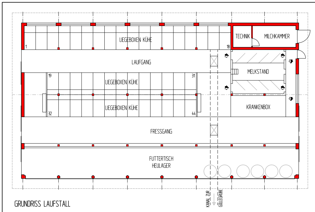
Abbildung 23: Laufstall (© Andreas Leichter)
