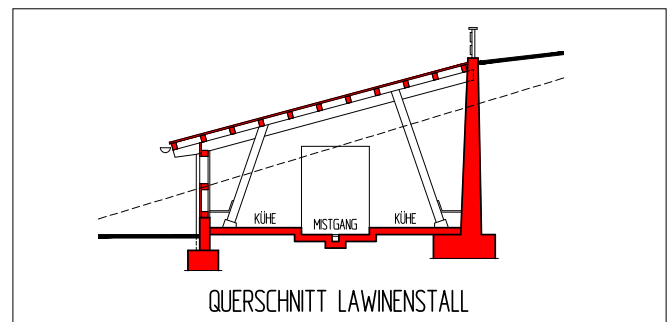
Abbildung 40: Querschnitt Lawinestall (© Andreas Leichter)
