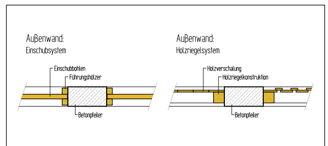
Abbildung 32: Stallwand mit massiven Pfeilern (© Andreas Leichter)
