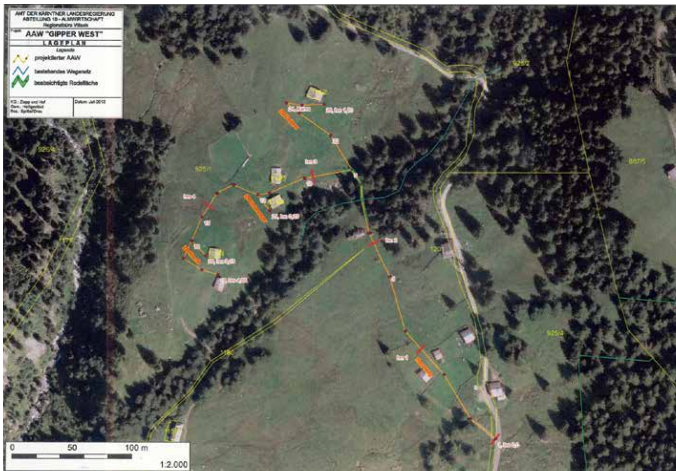
Abbildung 8: Lageplan mit Orthophoto – Darstellung der Grundstücksgrenzen und des Wegprojekts (© Friedrich Walter Merlin)
