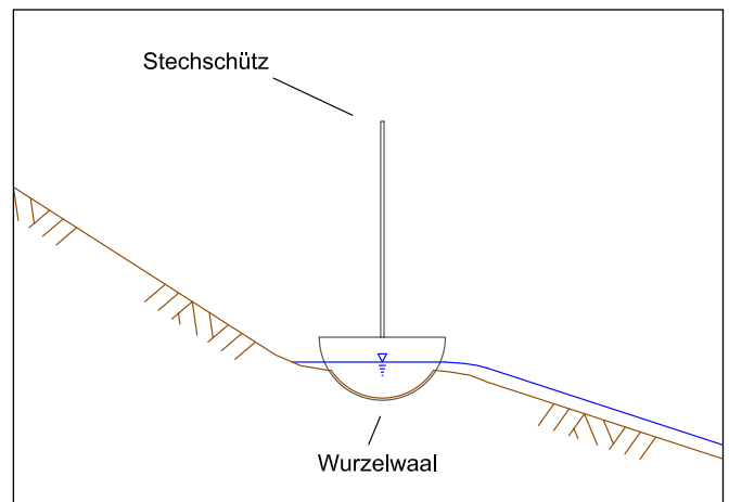
Abbildung 79: Verwendung eines Stechschützes oder Wassereisens (© Stefan Hellebart)
