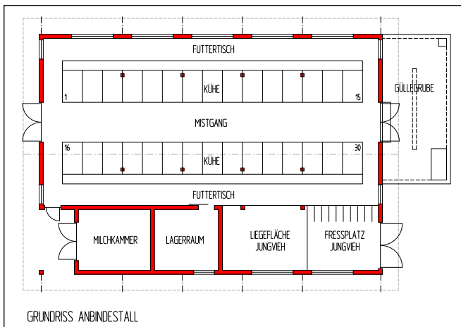
Abbildung 29: Grundriss Anbindestall (© Andreas Leichter)
