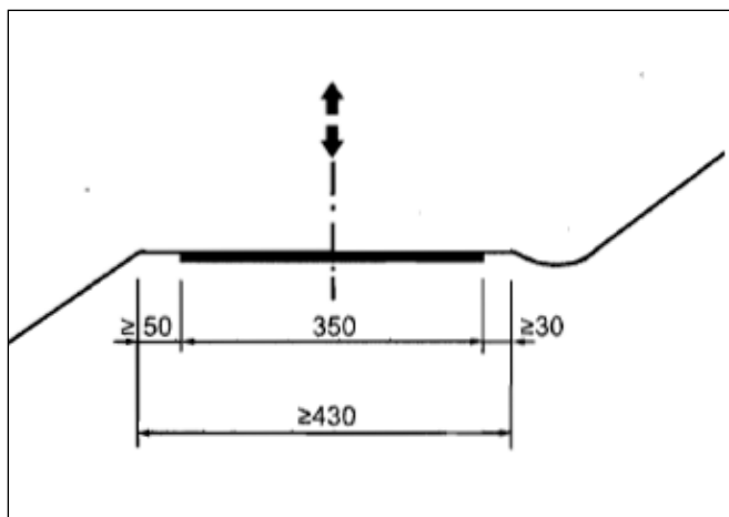
Abbildung 6: Regelquerschnitt L4 lt. RVS 03.03.81 (© RVS)
