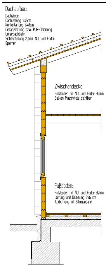
Abbildung 37: Fassadenschnitt Blockbau (© Andreas Leichter)
