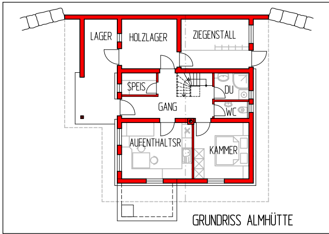
Abbildung 36: Grundriss Almhütte (© Andreas Leichter)
