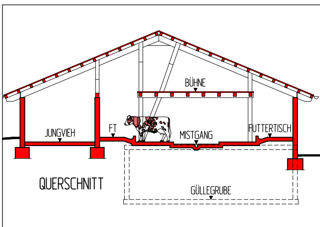
Abbildung 30: Querschnitt Anbindestall (© Andreas Leichter)
