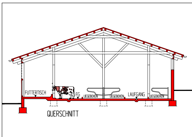
Abbildung 24: Querschnitt (© Andreas Leichter)
