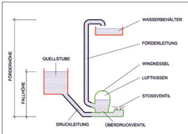
Abbildung 72: Schemaskizze zum Hydraulischen Widder (© Stefan Hellebart)
