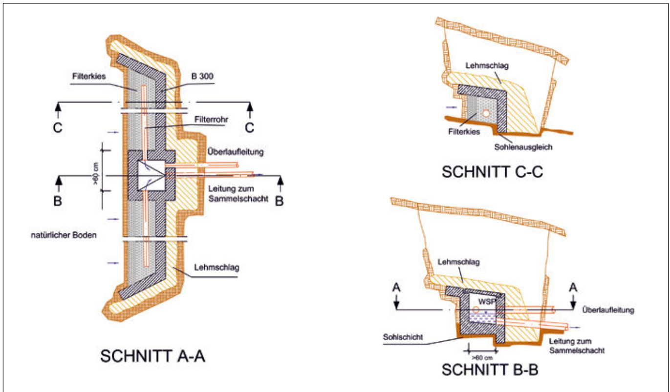
Abbildung 71: Schemaskizze einer Quellfassung nach DVGW (© Stefan Hellebart)
